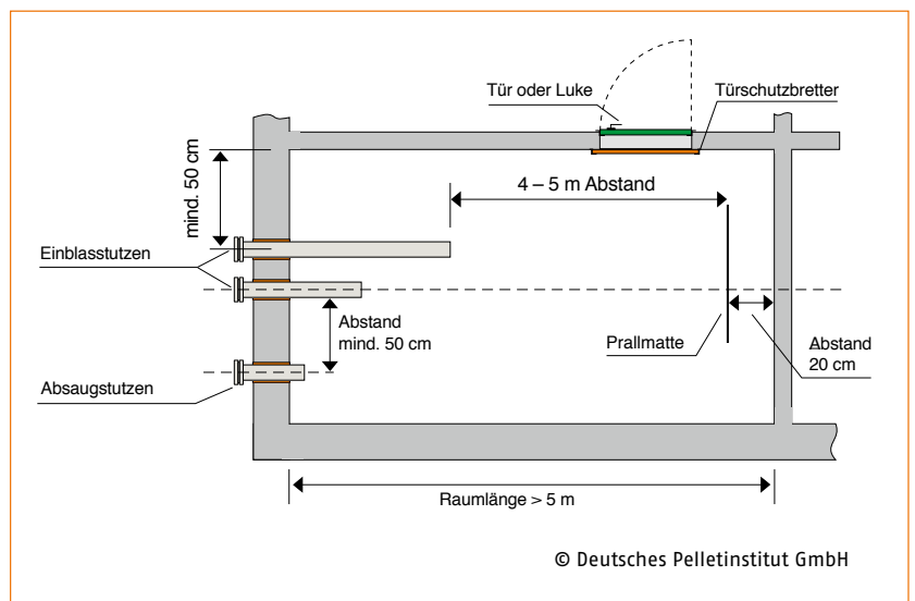
Abb. 25: Ausführungsbeispiel für lange Lagerräume (Draufsicht)
