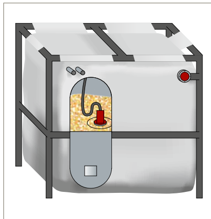
Abb. 11a: Flachbodensilo mit Saugentnahme von oben
