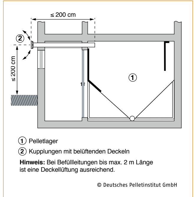
Abb. 29: Belüftungslösung für Pelletlager mit Befüllleitung ≤ 2 m
